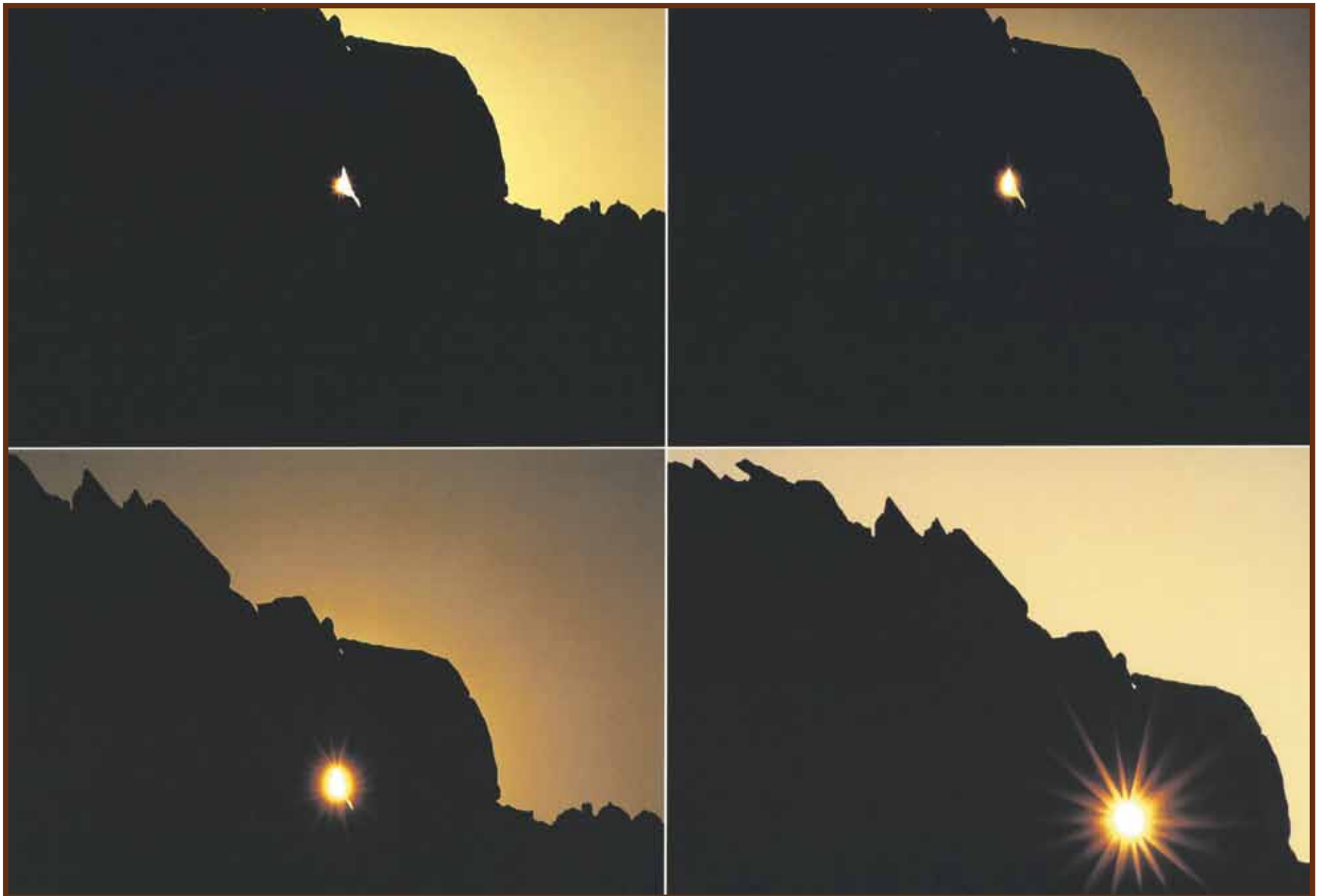
Imatges seqüencials del Sol quan penetra el Forat de la Coma, extretes del llibre El Pic d'Arcalís, la Muntanya Solar , firmades pel fotògraf Jaume Riba.
